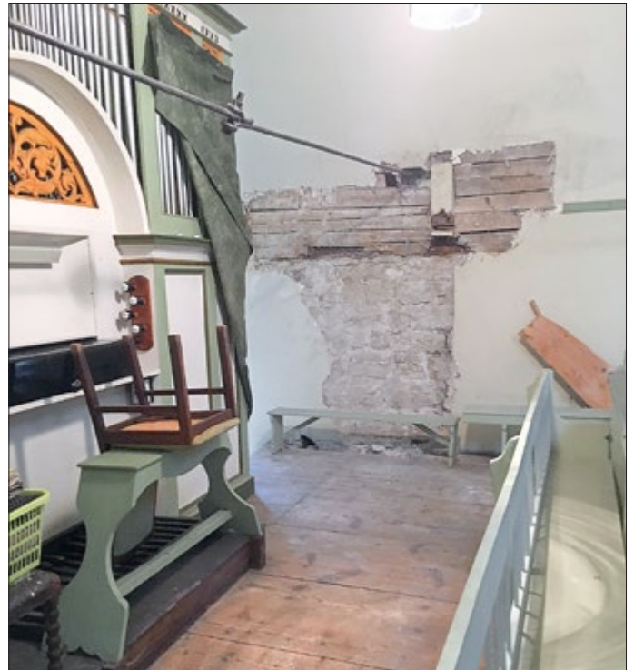
Schadstelle am Mauerwerk durch Pilzbefall
